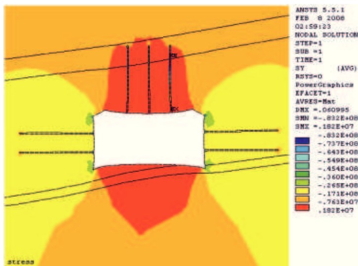
Рис. 6. Изменение и распределение максимальных напряжений в зонах, окружающих горную выработку: а и б – характер изменения и этюра (при \alpha = 10^\circ ) максимальных нормальных напряжении
